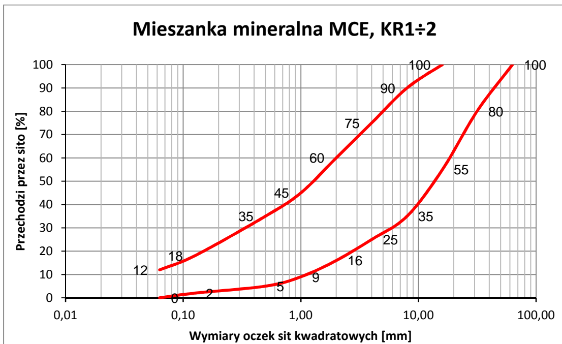
Rysunek 5.1. Uziarnienie mieszanki mineralnej MCE dla ruchu KR1÷KR2
